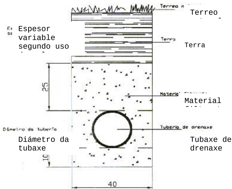
Gabia para a colocación de tubaxe de drenaxe
